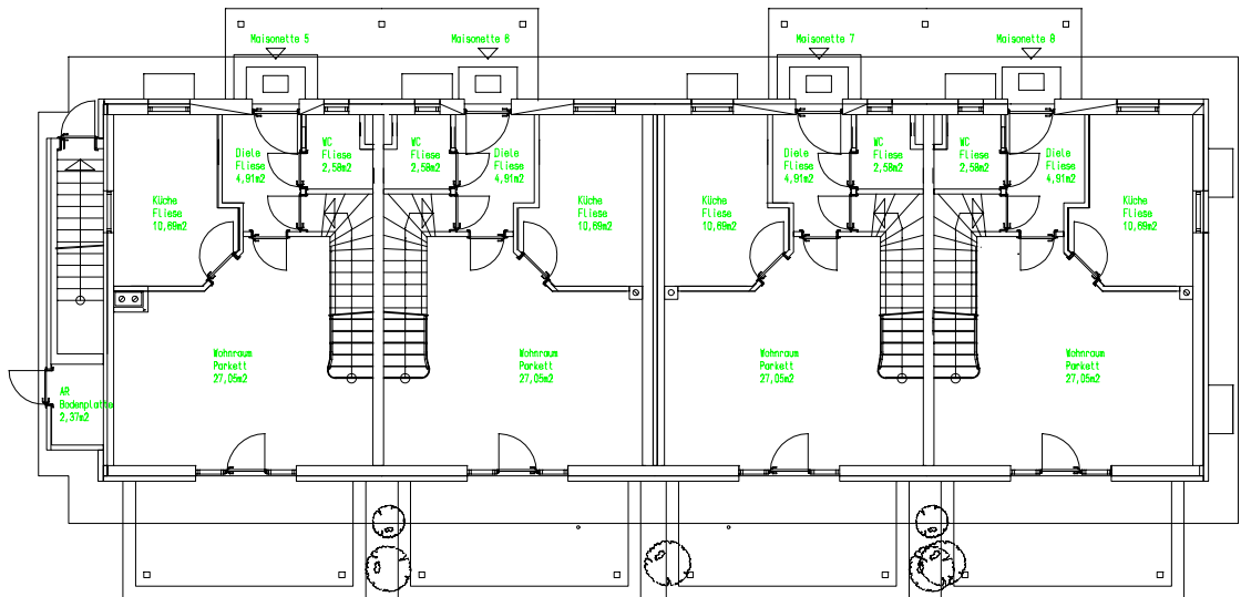
WA ADMONT EG MAISONNETTE 5-8
